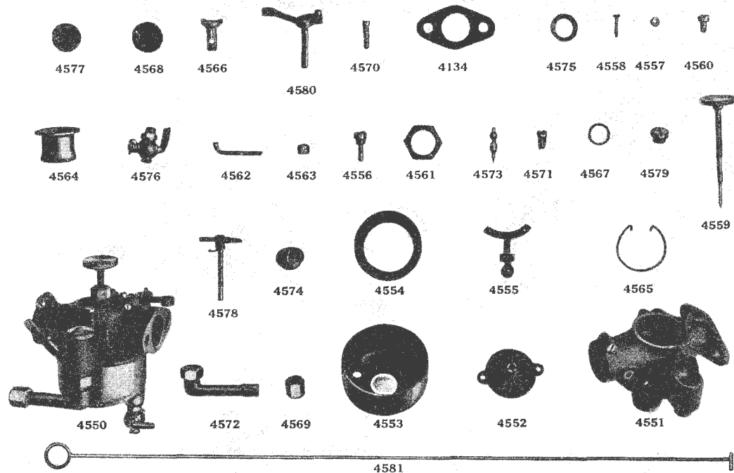
Plate No. 15—1912 Holley Carburetor Parts
