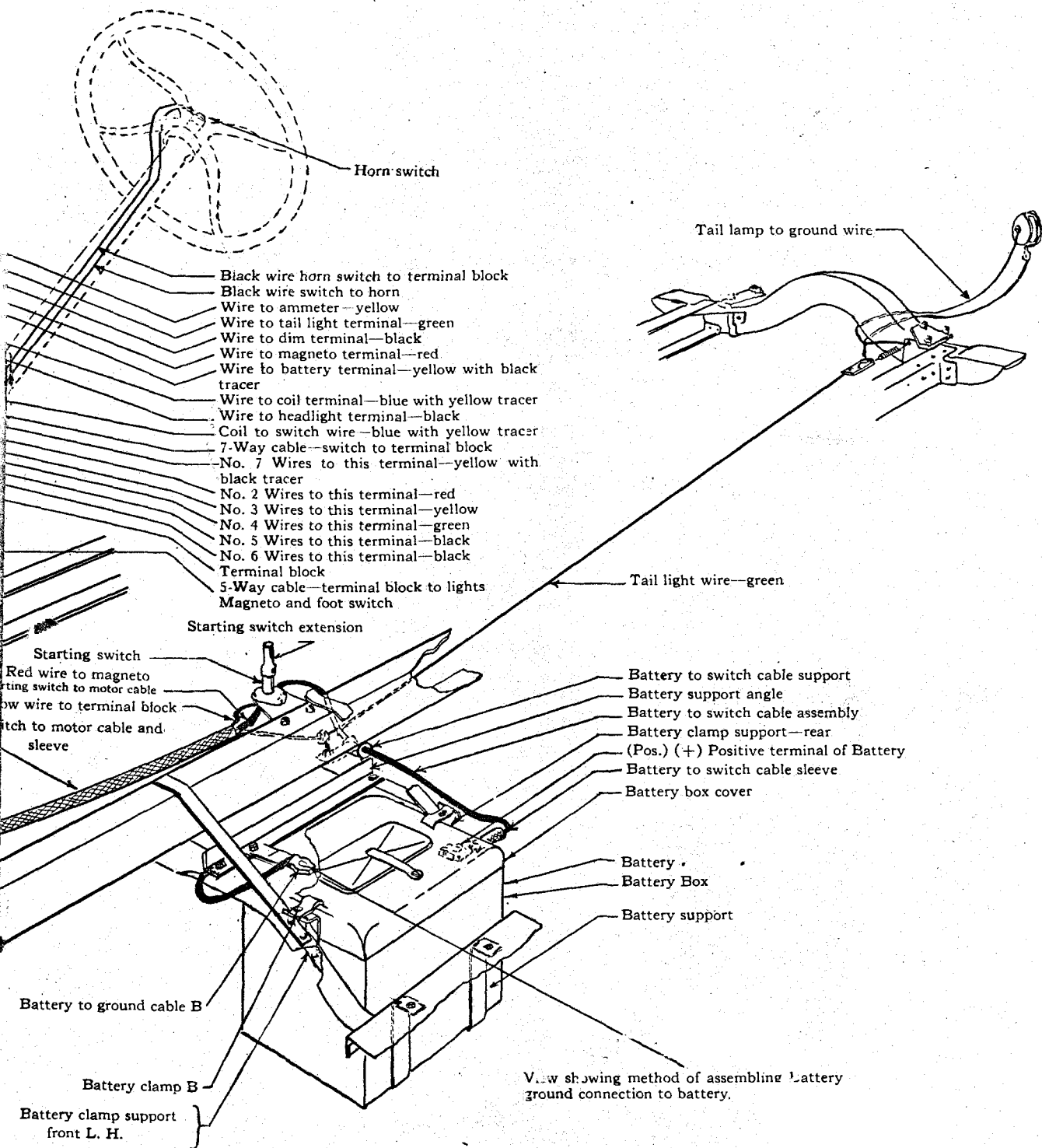
WIRING DIAGRAM T T CHASSIS L. H. C.
